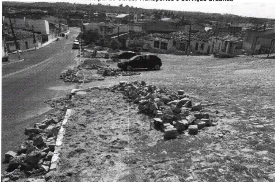
SERVIÇO DE RECUPERAÇÃO NA LADEIRA DO MERCADO MERCANTE
