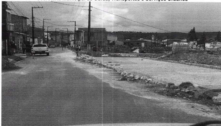
PAVIMENTAÇÃO CONCLUÍDA DO ESTACIONAMENTO DO MIRANTE
