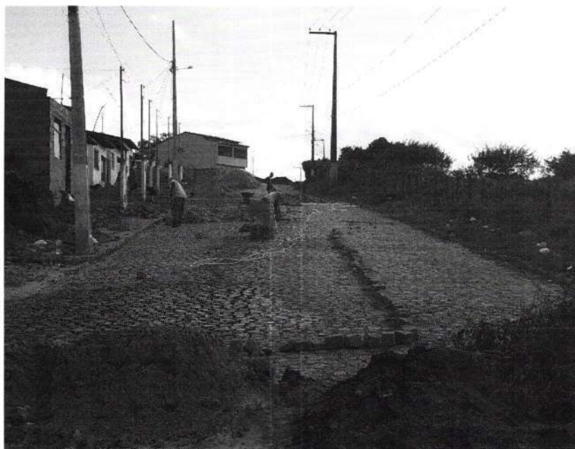
SERVIÇO DE PAVIMENTAÇÃO NA "LADEIRA DE SILVEIRA"
