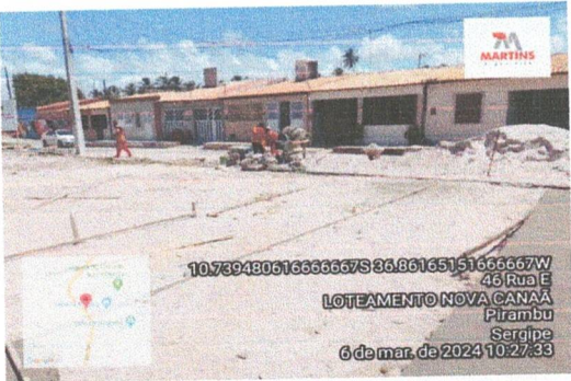
Colchão de areia, regularização de piso e piso em concreto
