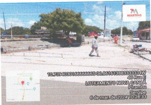
Colchão de areia, regularização de piso e piso em concreto
