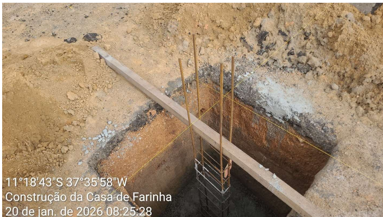
Sapatas de concreto armado
